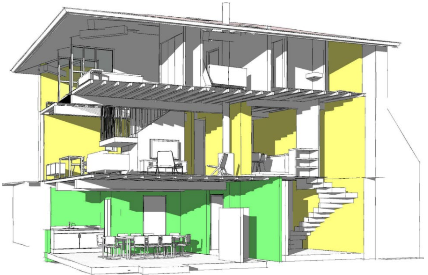
Vue en coupe de la maison depuis la rue
